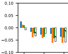
Beta-NSE
