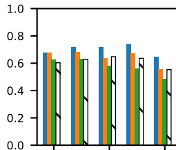
KGE
