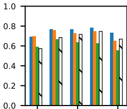
NSE
