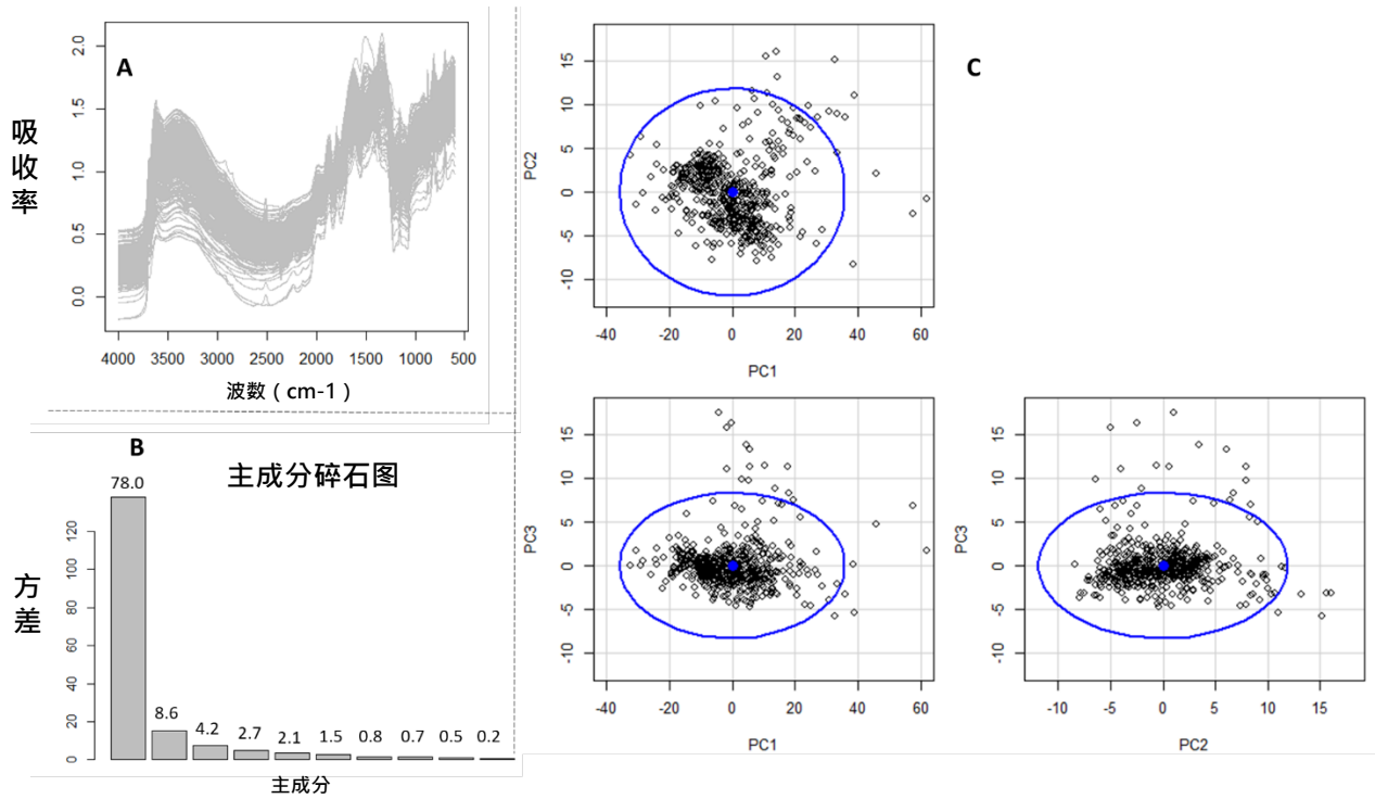
图5 MIR光谱数据主成分分析示意图: (A) 在光谱空间的土壤MIR光谱; (B) 前10个主成分的碎石图及其解释总体变异的百分比; (C) 前三个主成分的两两散点图。
