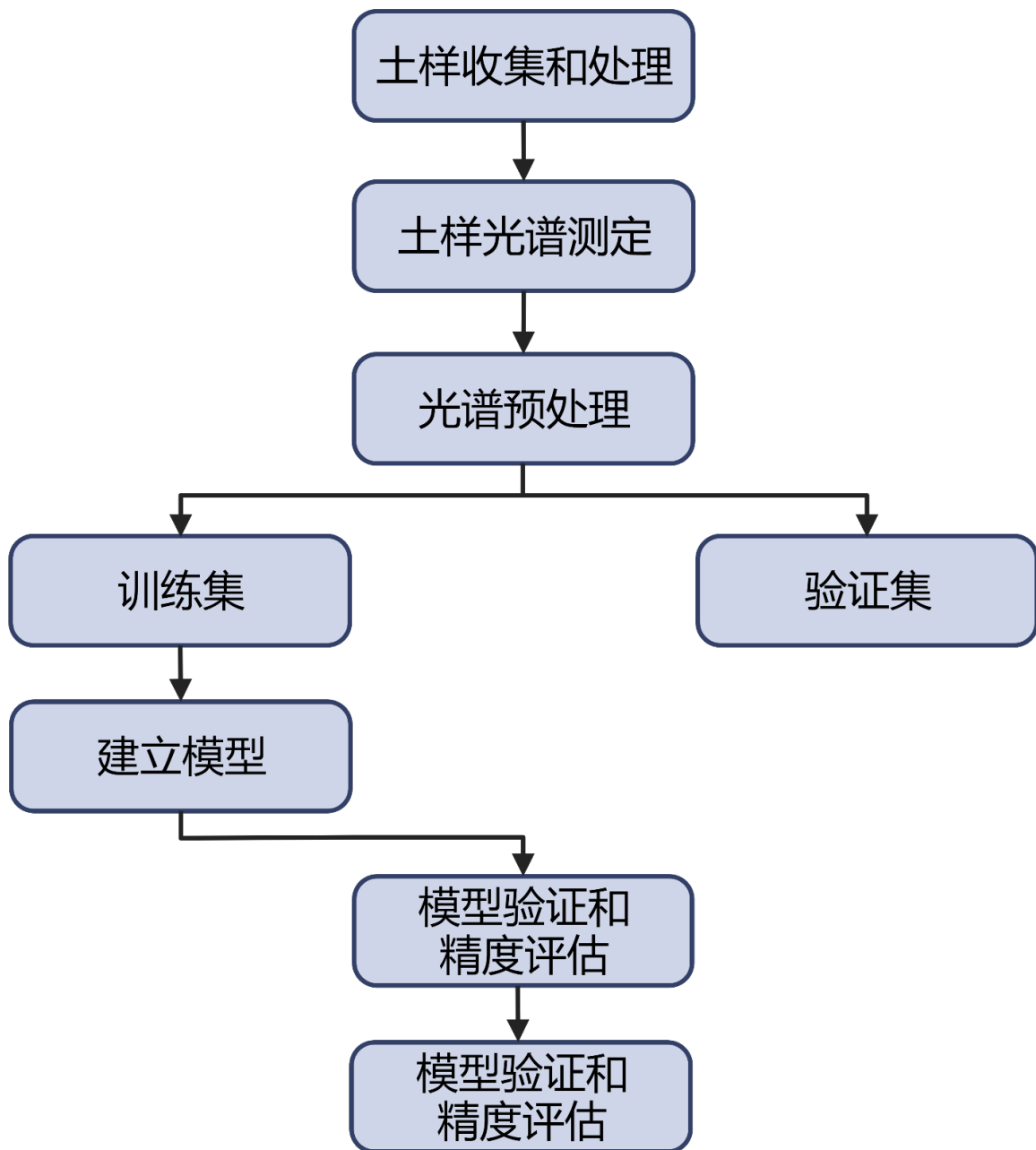
图2 Vis-NIR和MIR光谱分析的流程。
