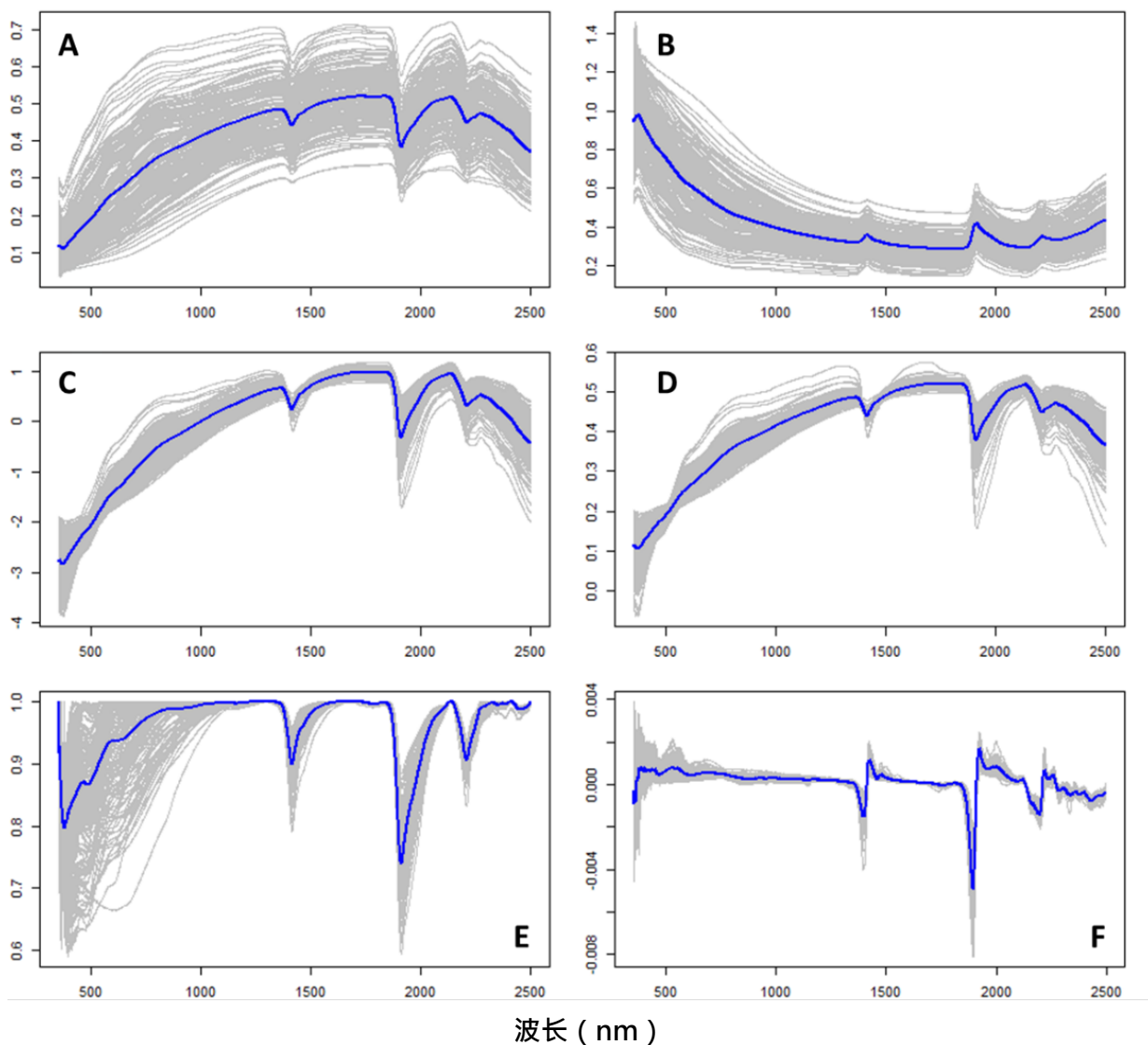
图3 示例数据中的vis-NIR光谱 ( n=201 ) 经不同预处理后的结果: (A) 原始反射光谱; (B) 吸收光谱; (C) 标准正态变换光谱; (D) 多元散射校正光谱; (E) 连续统去除光谱; (F) SG滤波加一阶导光谱。蓝色曲线代表平均光谱。
