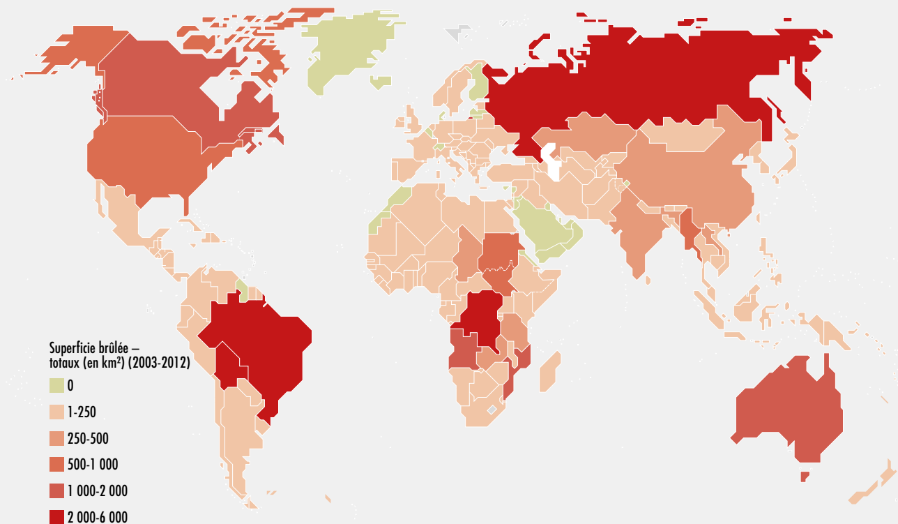
FIGURE 22 SUPERFICIE FORESTIÈRE BRÛLÉE
