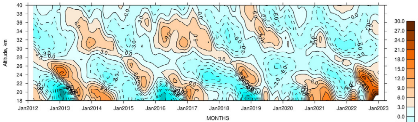
Aura-MLS v5 Ozone [%], 5S-5N
