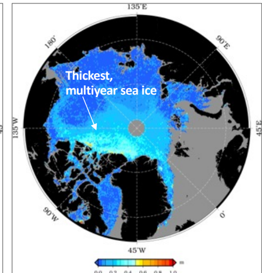
ESA CryoSat-2
