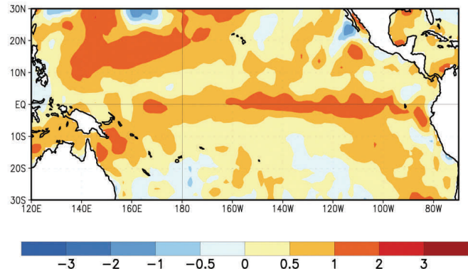
SST Anomalies (°C)
